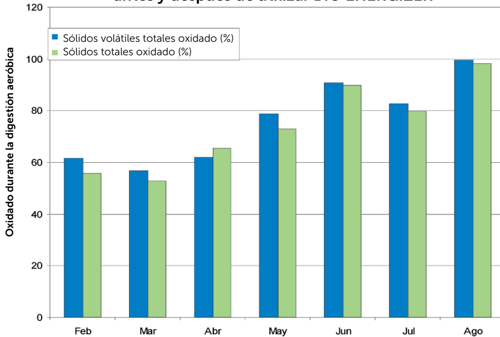
Efficiencia de la destrucción de sólidos volátiles antes y después de utilizar BIO ENERGIZER®
